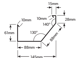
SHORELINE® Mini Gutter 300 Girth
